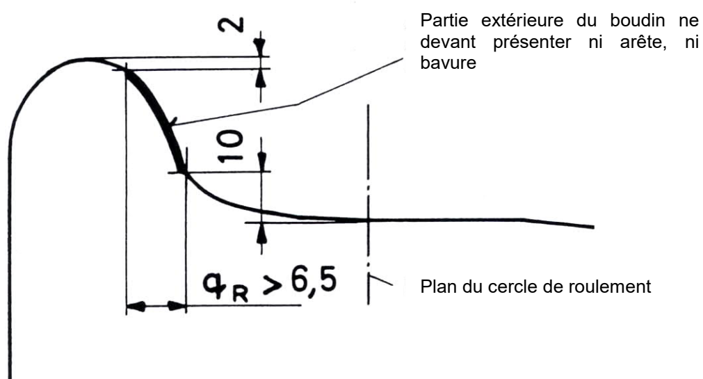
Figure 1 Profil admissible la partie extérieure du boudin
