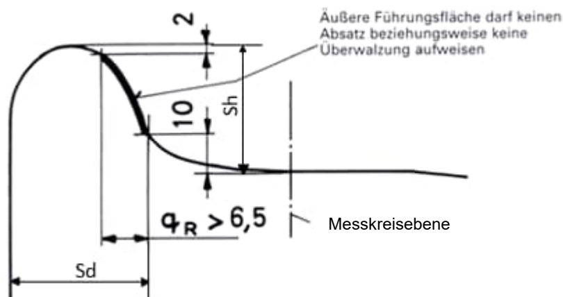
Bild 2: Abmessungen einer Rad-Kombi-Prüflehre für die Prüfung der Masse q_R , S_d , S_h inkl. Überwalzung und Hohllauf
