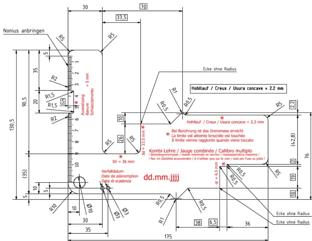
Bild 2: Abmessungen einer Rad-Kombi-Prüflehre für die Prüfung der Masse q_R , S_d , S_h inkl. Überwalzung und Hohllauf
