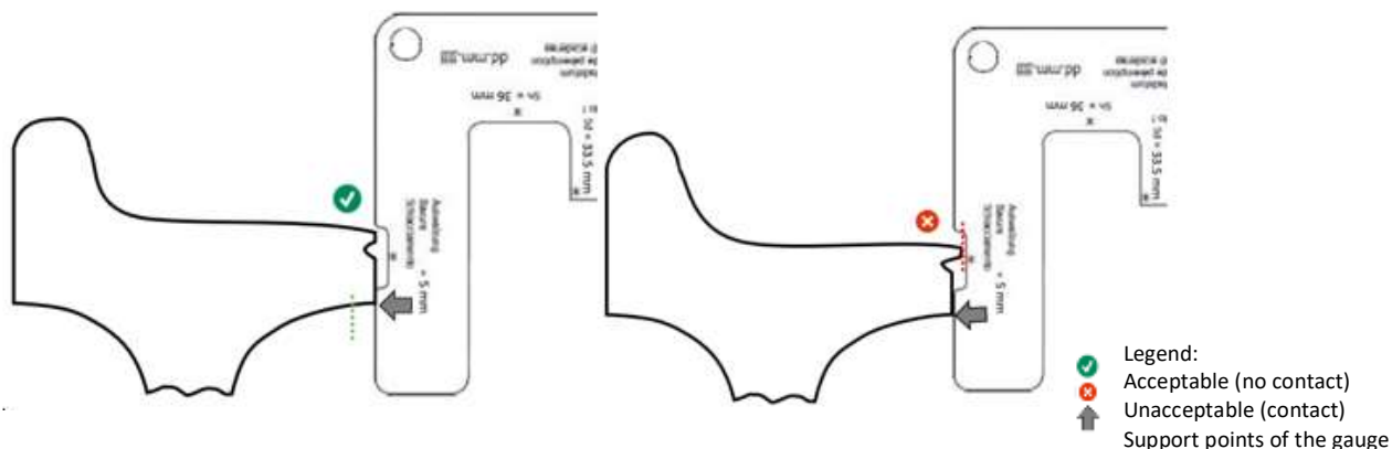
Fig. 8 – False flange
