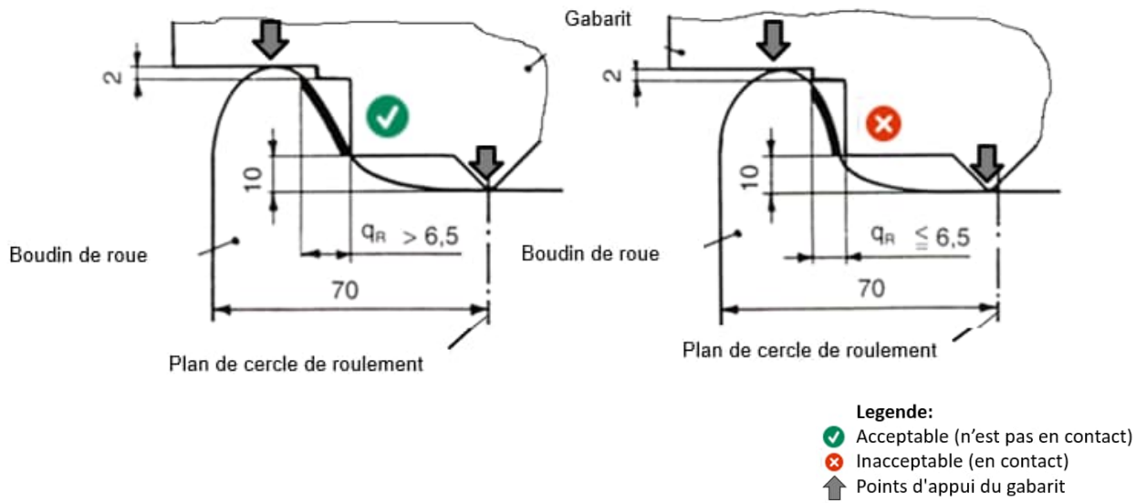
Figure 4 : Boudin de roue avec arêtes vives ou formation de bavures
