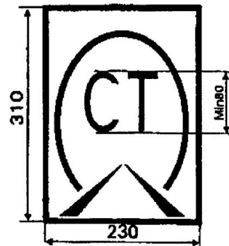
Bild 2 In Großbritannien (Infrastruktur NETWORK RAIL) zugelassene Wagen, die den Ärmelkanaltunnel benutzen
