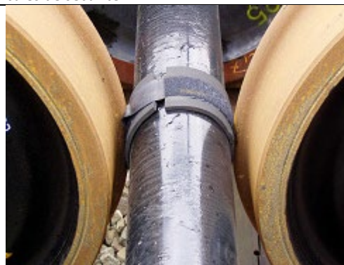
Photo 4 : Stockage en quinconce sur voie avec protection de contact
